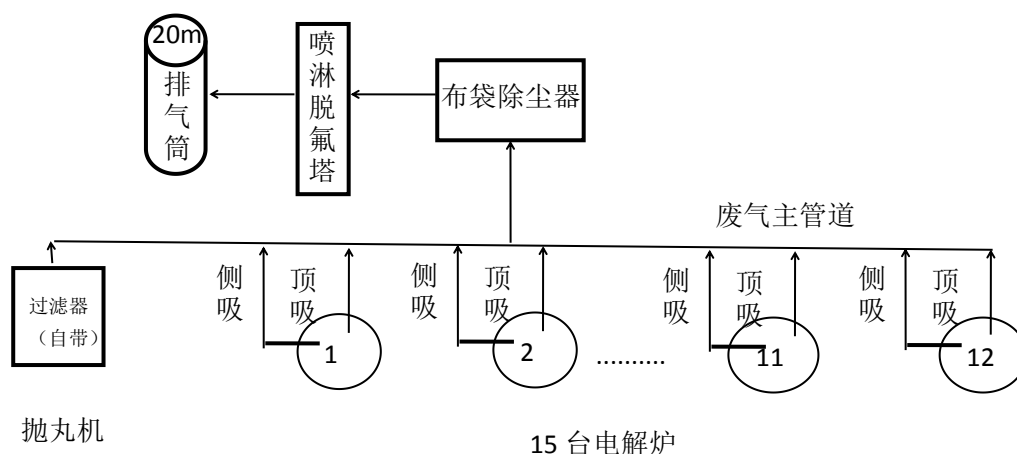
图 3-5 本项目电解废气走向工艺流程图
