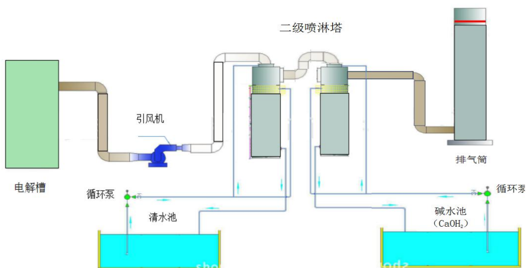
图 3-4 本项目喷淋脱氟装置工艺流程
