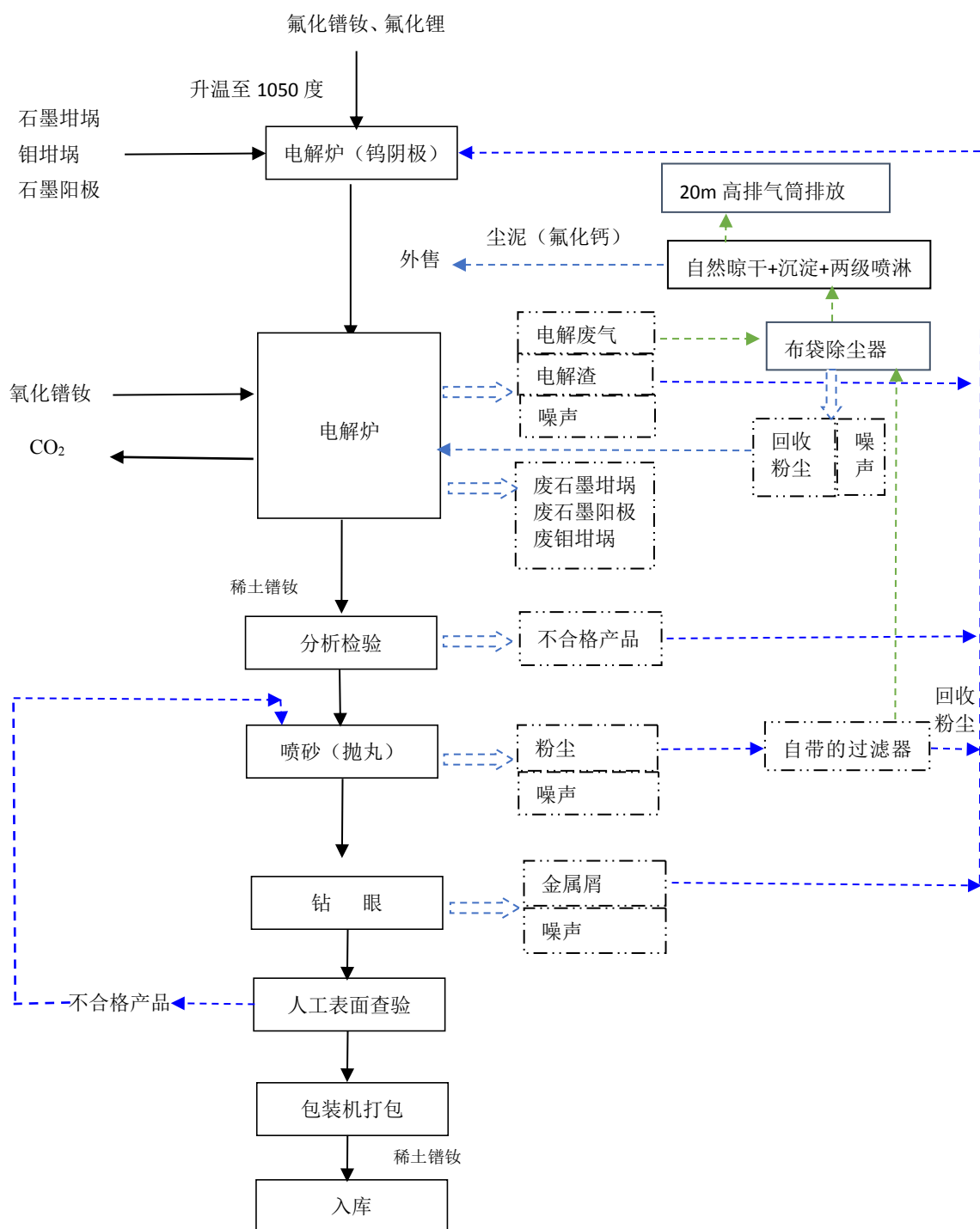
图 3-3 本项目稀土镨钕生产工艺流程及污染环节图
