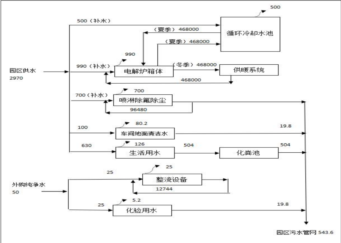
图 3-1 本项目水平衡图（单位 t/a）
